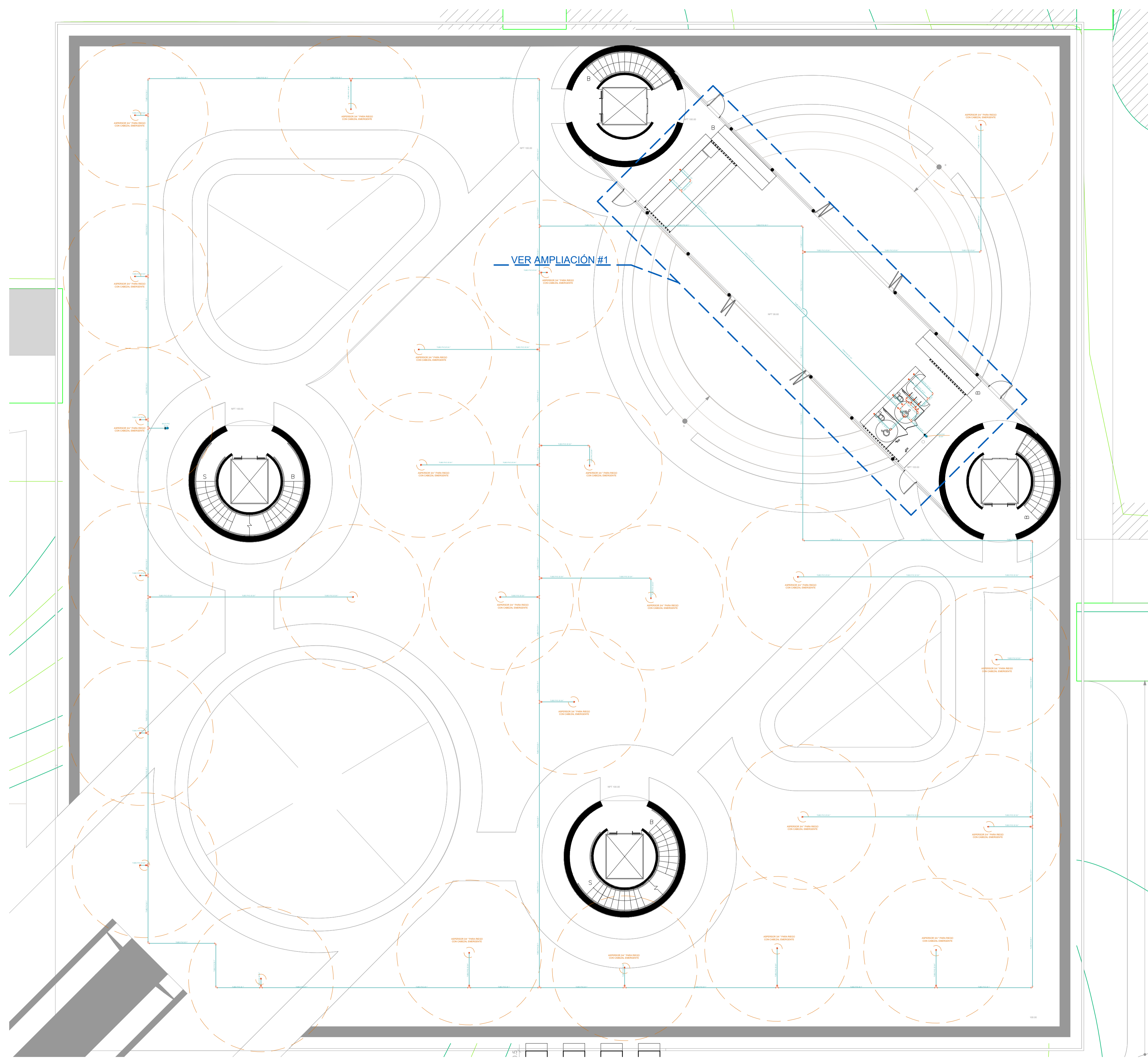
PLANO DE AGUA POTABLE TERRAZA ESCALA 1 : 150
